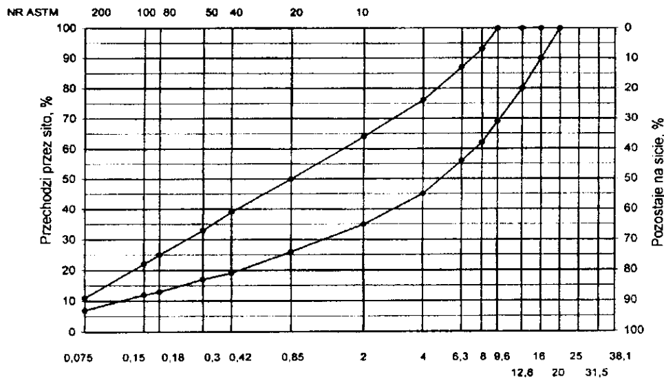
Rys. 2. Krzywe graniczne uziarnienia mieszanki mineralnej BA od 0 do 16mm, od 0 do 12,8 mm do warstwy ścieralnej nawierzchni drogi o obciążeniu ruchem KRI lub KR2
