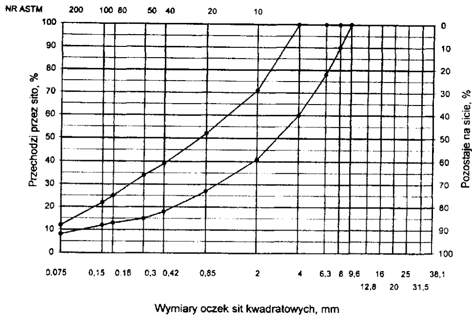
Rys. 3. Krzywe graniczne uziarnienia mieszanki mineralnej BA od 0 do 8mm, od 0 do 6,3 mm do warstwy ścieralnej nawierzchni drogi o obciążeniu ruchem nawierzchni drogi o obciążeniu ruchem KRI lub KR2
